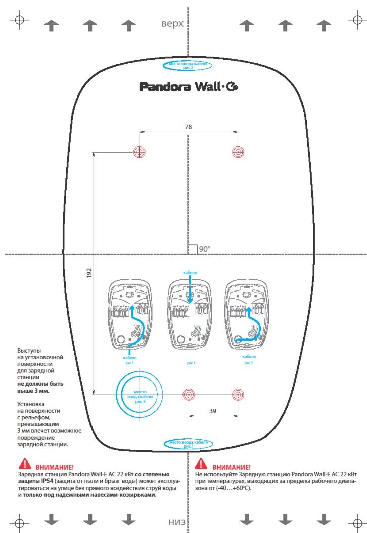
Рисунок 3. Разметка крепежа
